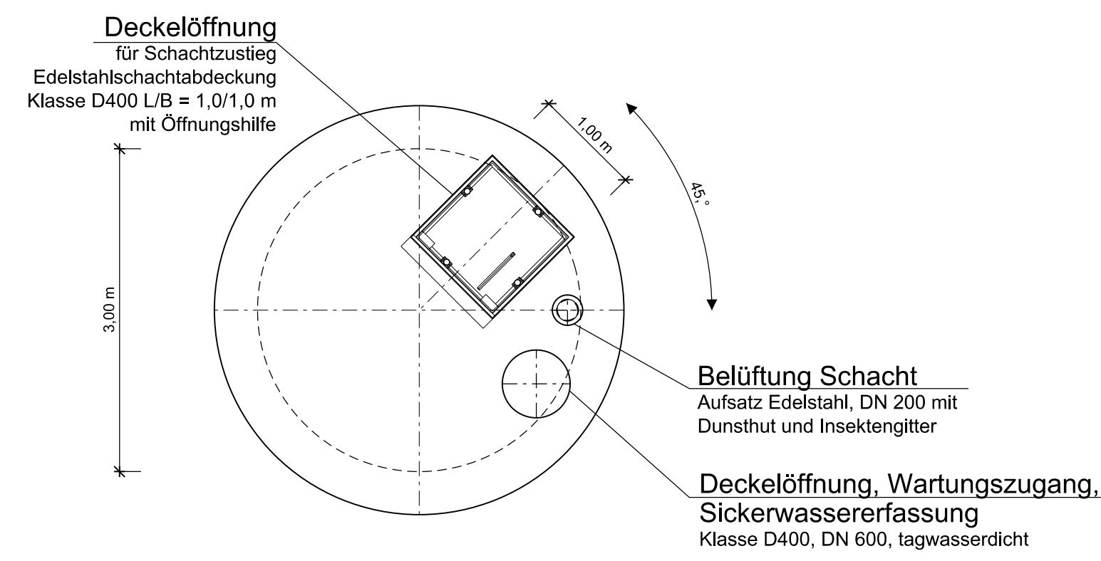
Draufsicht (Schachtdeckel)
