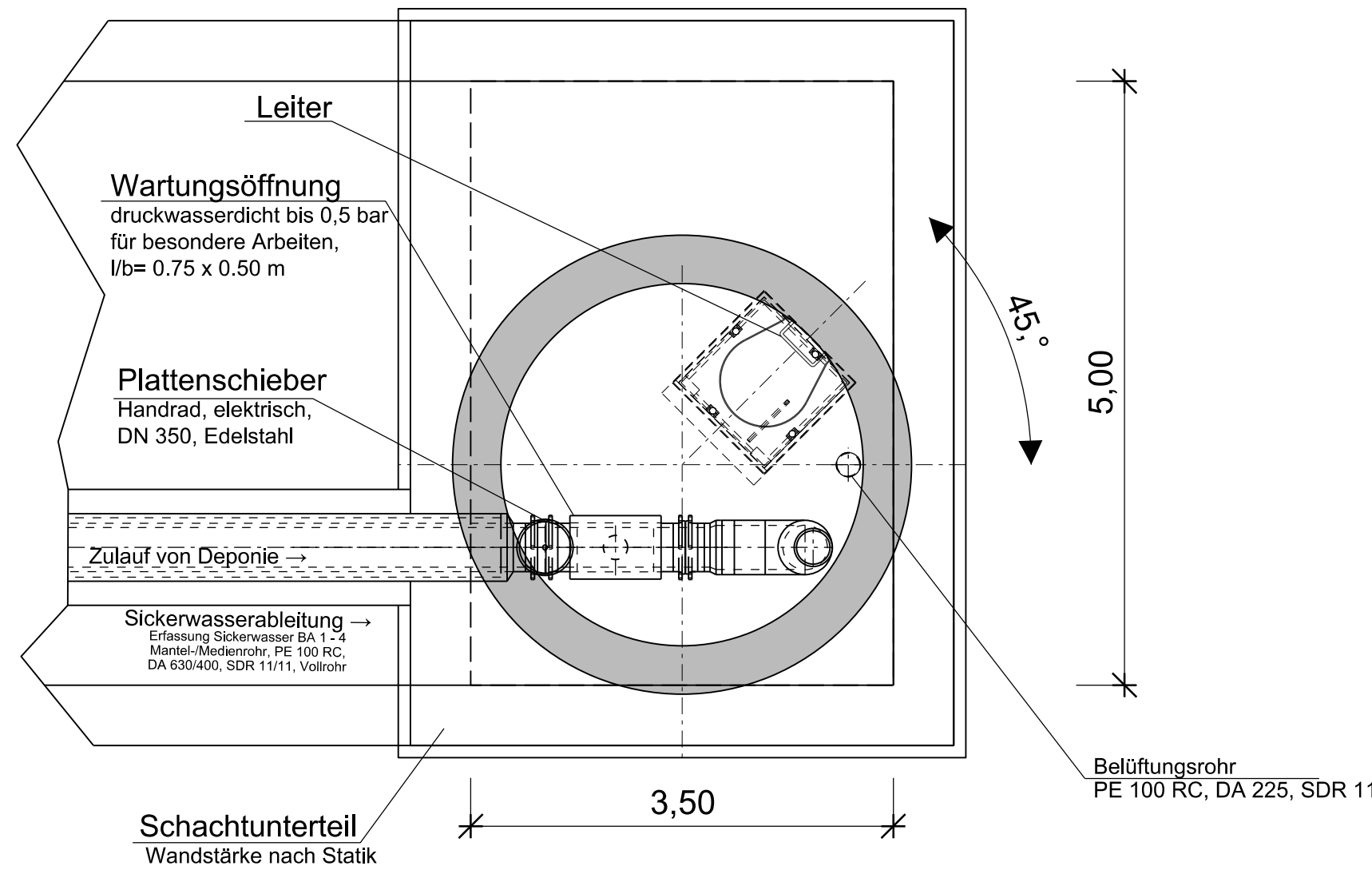
Schnitt D - D (schematisch dargestellt)
