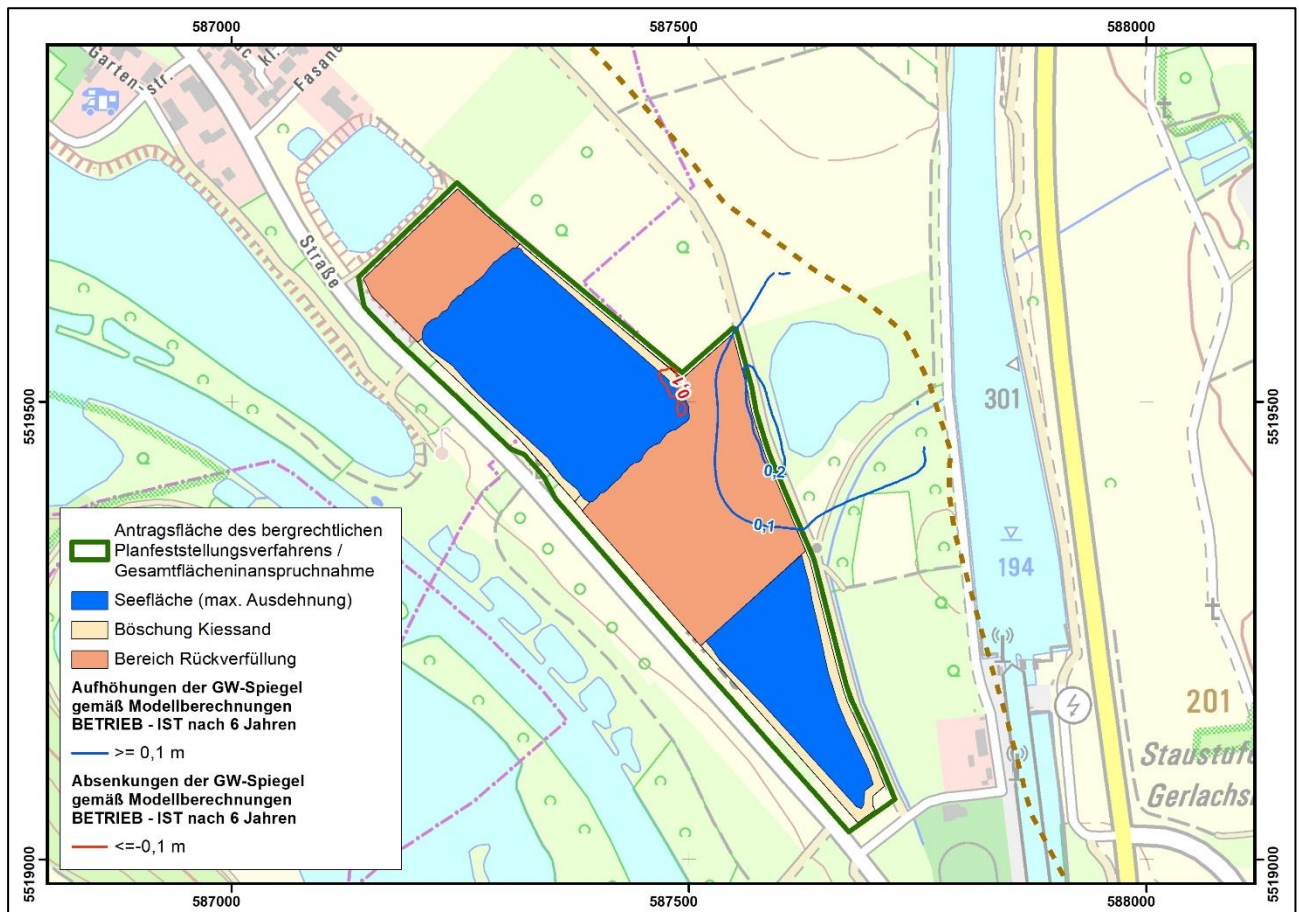
Abbildung 3-3: Modellberechnung Differenzenplan BETRIEB – IST-Zustand aus /22/
