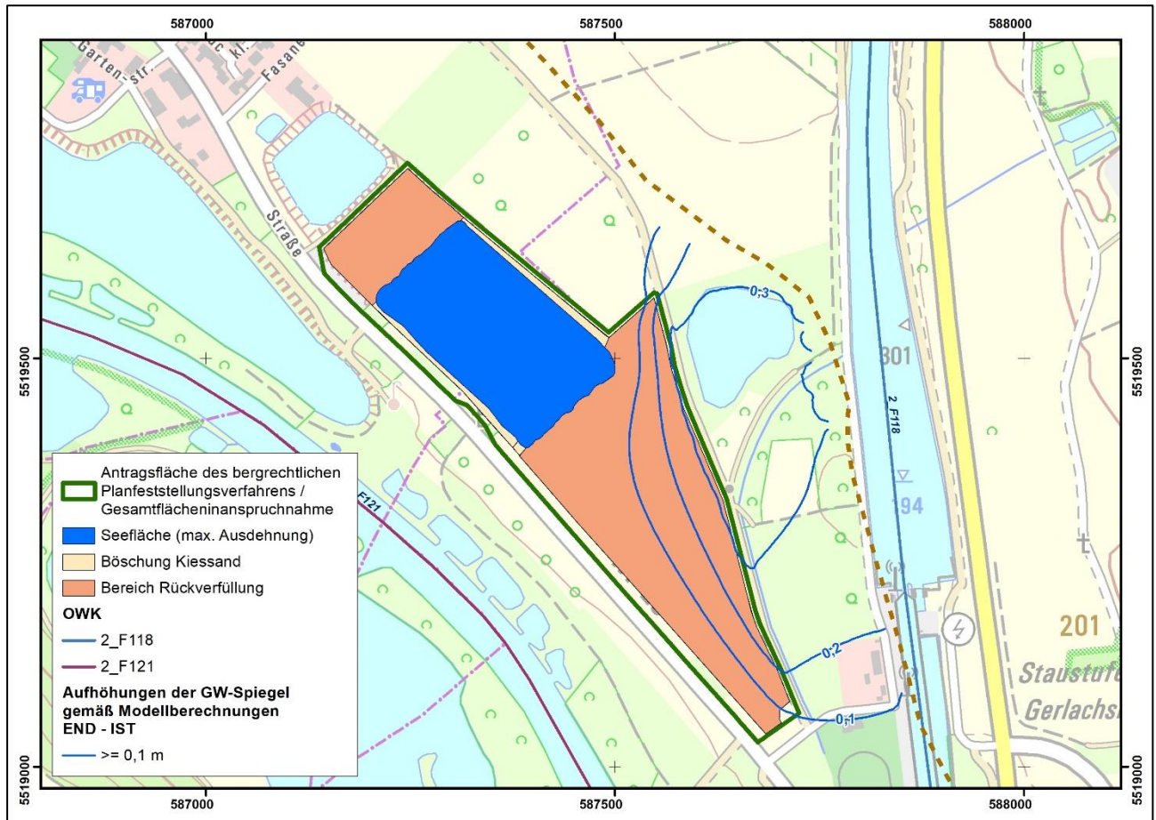
Abbildung 3-4: Modellberechnung Differenzenplan END – IST-Zustand aus /22/
