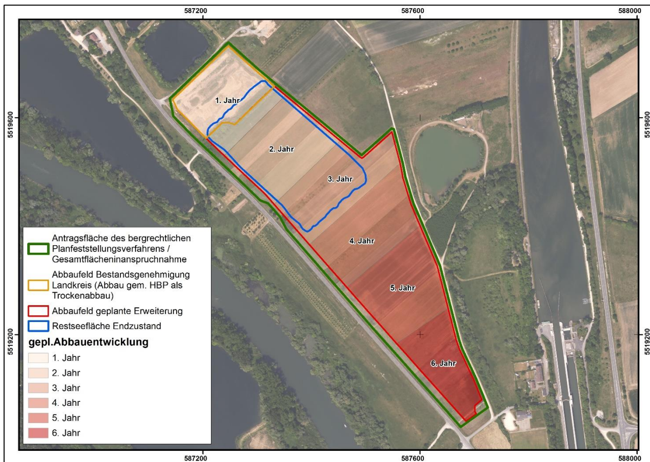
Abbildung 3-2: Abbauplanung Vorhaben Kiesabbau Sommerach
