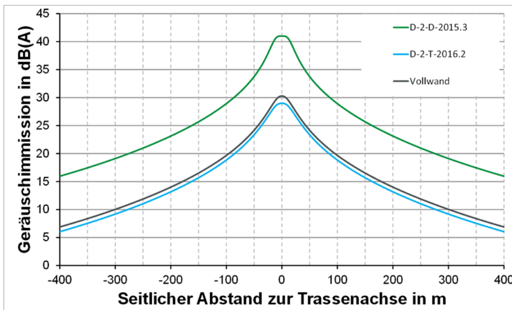
Abbildung 12: Berechnete Geräuschimmission in Abhängigkeit vom seitlichen Abstand zur Trassenachse für die Masttypen Stahlgitter-Donau, Stahlgitter-Tonne und Vollwand-Tonne
