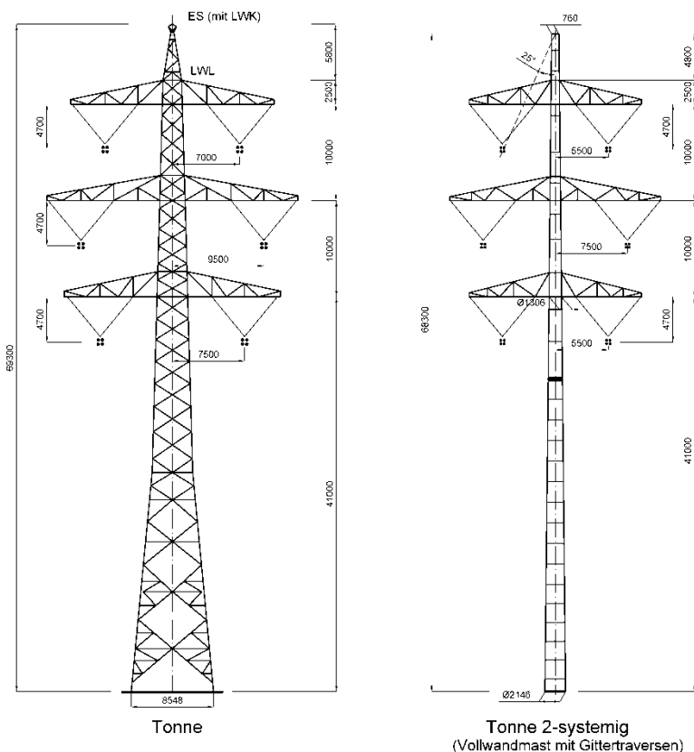
Abbildung 7: Gegenüberstellung von Stahlgitter – und Vollwandbauweise für einen 2-systemigen Mast in Tonnenkonfiguration
