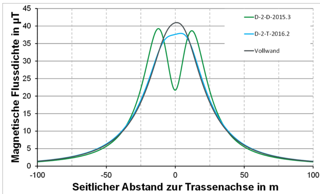
Abbildung 11: Berechnete magnetische Flussdichte in Abhängigkeit vom seitlichen Abstand zur Trassenachse für die Masttypen Stahlgitter-Donau, Stahlgitter-Tonne und Vollwand-Tonne
