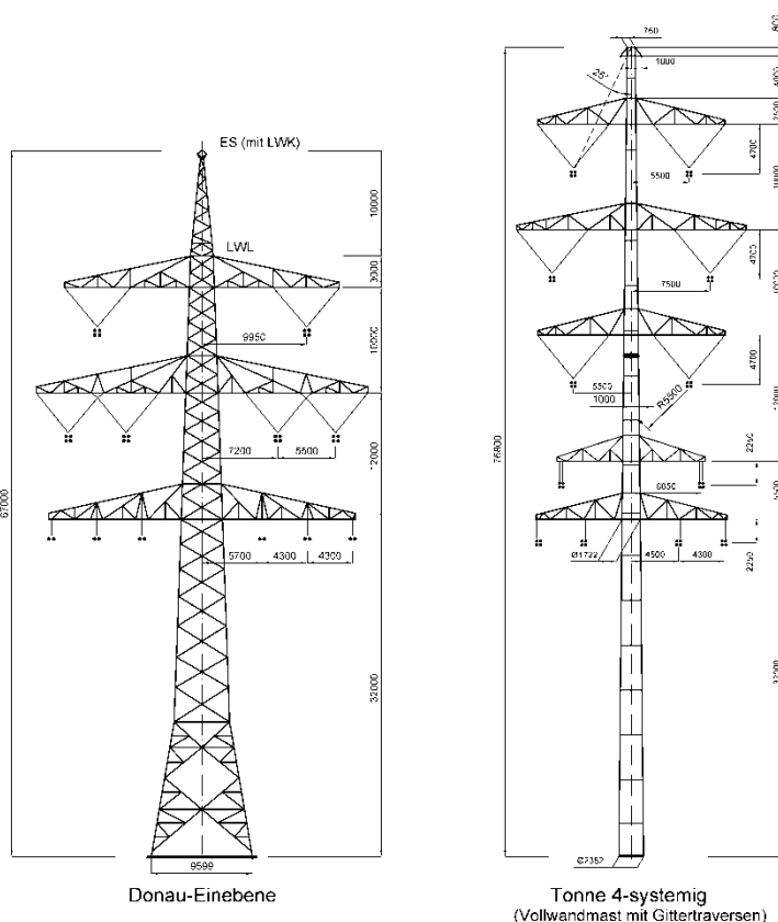
Abbildung 9: Gegenüberstellung von Stahlgitter – und Vollwandbauweise für einen 4-systemigen Mast (110-kV-Mitnahme)
