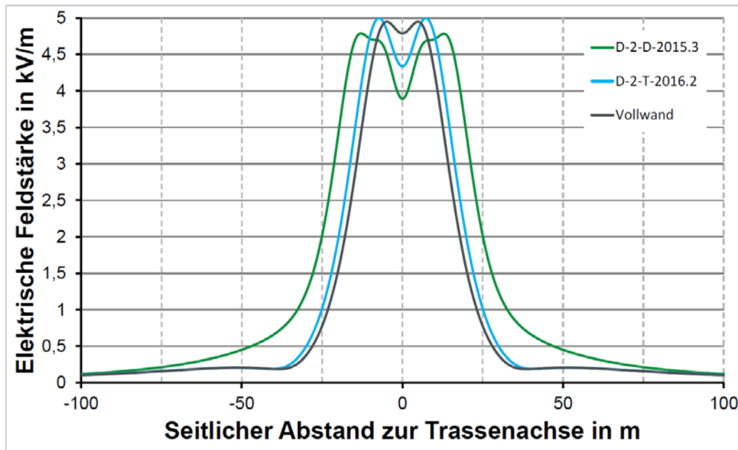
Abbildung 10: Berechnete elektrische Feldstärke in Abhängigkeit vom seitlichen Abstand zur Trassenachse für die Masttypen Stahlgitter-Donau, Stahlgitter-Tonne und Vollwand-Tonne
