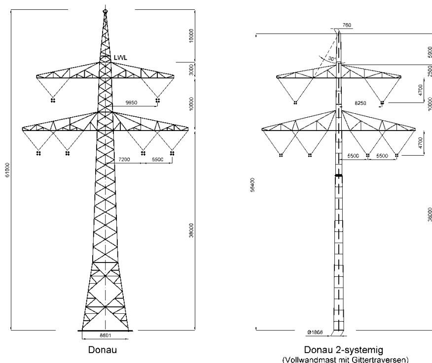
Abbildung 8: Gegenüberstellung von Stahlgitter – und Vollwandbauweise für einen 2-systemigen Mast in Donaukonfiguration
