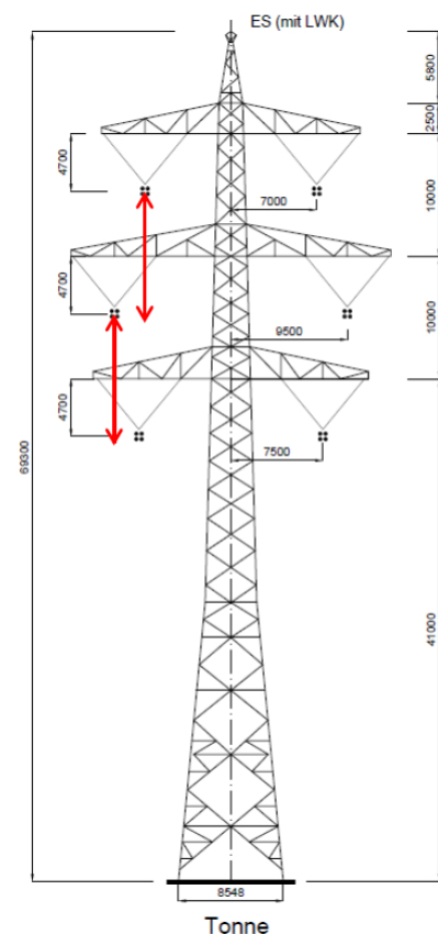
Abbildung 3: Horizontaler Phasenversatz
