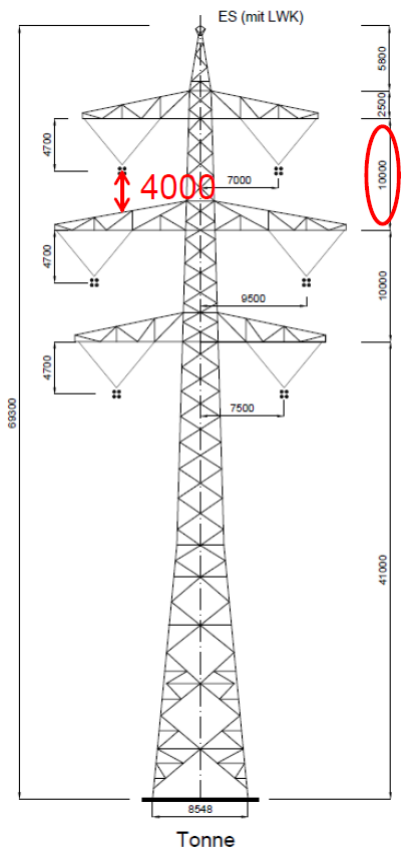
Abbildung 2: Abstand Obergurt Traverse zur darüber liegenden Phase und Stockwerksabstand
